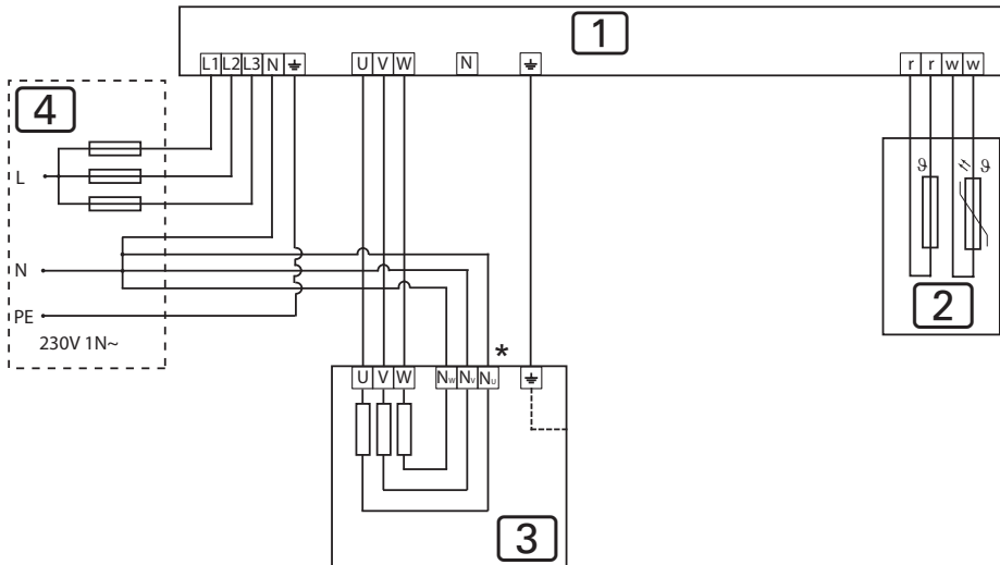
Bild 7 Anschlussplan 230V 1N~ Home fin 4,5 kW, 6,0 kW, 7,5 kW och 9,0 kW (HOME-F45 / HOME-F60 / HOME-F75 / HOME-F90)
